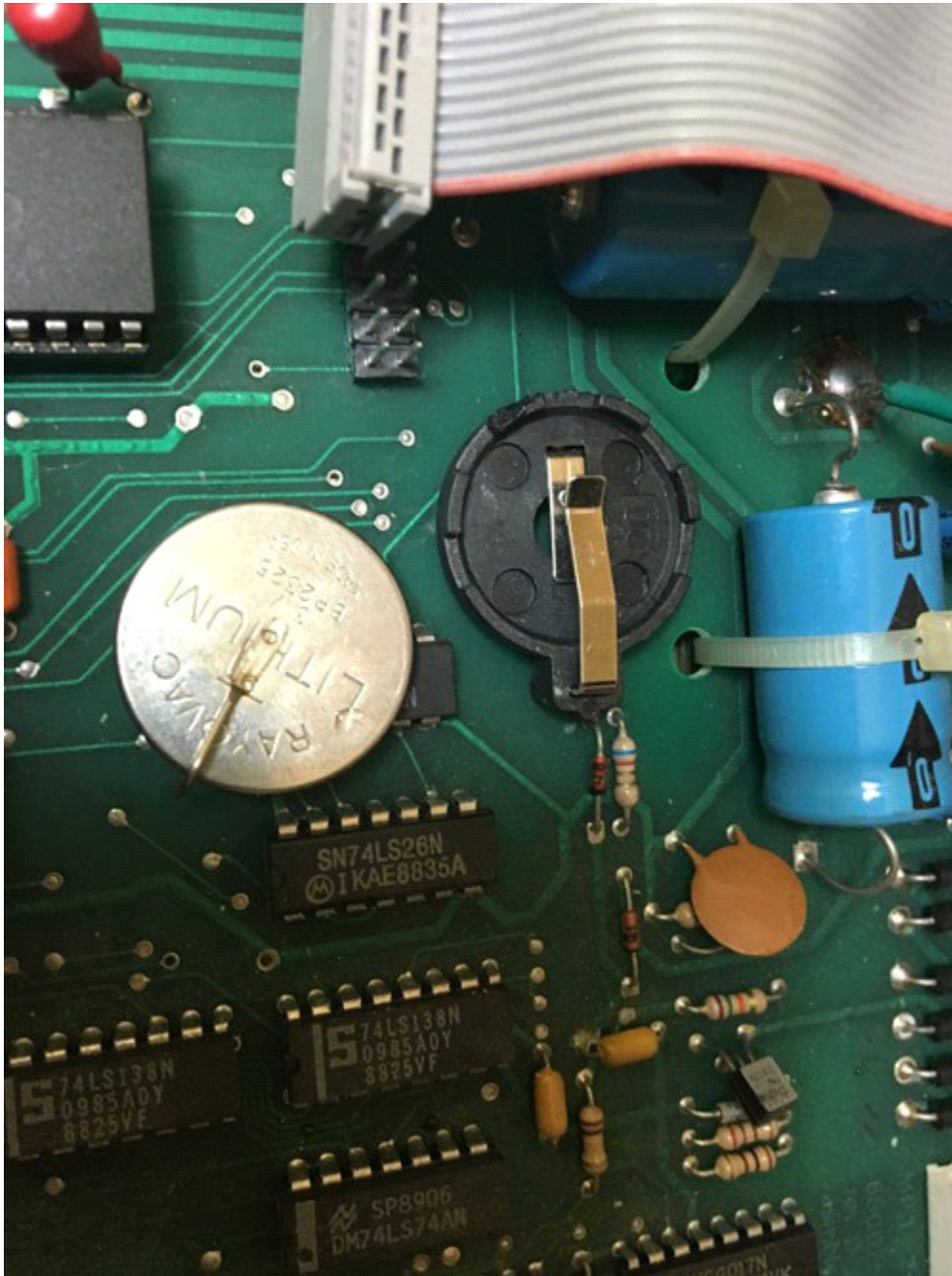
左 古い基盤直付けの電池 右電池ホルダー
